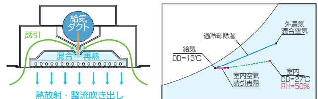
結露を防ぎ、優しい温度に整える誘引再熱と熱移動のイメージ
