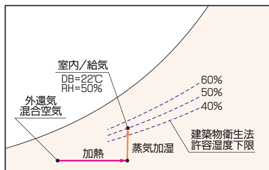
蒸気加湿
