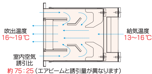
構造図
