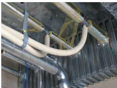
<本管側>
