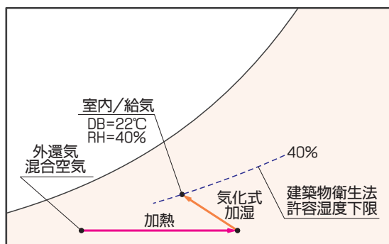
気化式加湿
