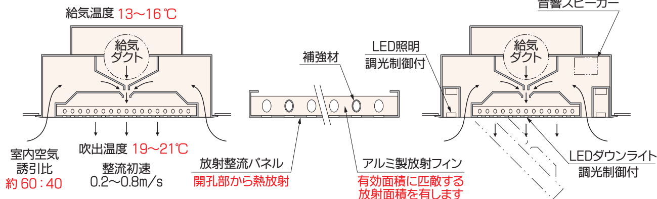
構造図
