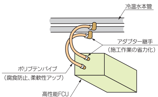
<枝配管>
