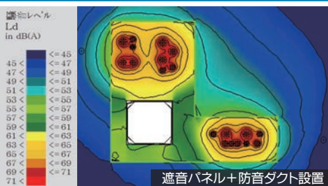
ビル屋上設置室外機の騒音解析例
