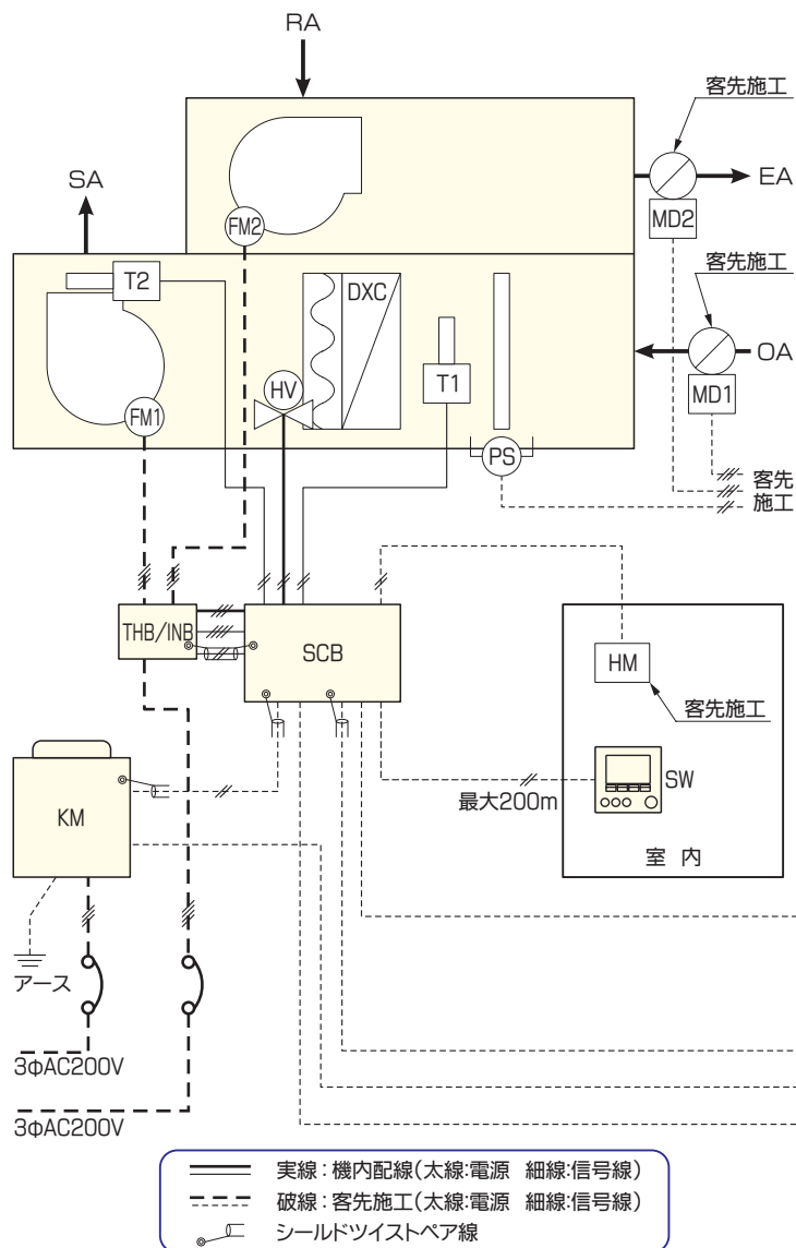
番号 名 称 備 考 1 外部加湿入力 無電圧a接点 ON:加湿 OFF:加湿停止 2 冷暖房モード切換入力 無電圧a接点 ON:冷房 OFF:暖房 3 遠方/手元切換入力 無電圧a接点 ON:遠方 OFF:手元 4 発停入力 無電圧パルスまたはレベル信号 5 送風入力 無電圧a接点 ON:送風 OFF:通常 6 運転状態出力 無電圧a接点 7 異常出力 無電圧a接点 8 送風機運転出力 無電圧a接点 9 冷房モード出力 無電圧a接点 10 暖房モード出力 無電圧a接点 11 除霜運転出力 無電圧a接点 12 3線式発停入力 無電圧または有電圧(DC24V) 13 非常停止入力 無電圧a接点 ON:通常 OFF:非常停止 OP1 風量制御入力 DC0~10V(4~10V=40~100%) OP2 商用切換入力 無電圧a接点 ON:商用 OFF:インバータ OP3 デマンド入力 無電圧a接点
