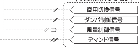
制御盤 オプション入出力仕様表
