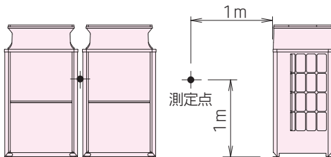
KM-24A
