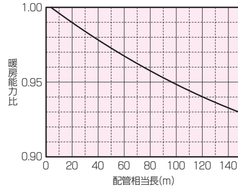
<暖房配管長補正線図>
