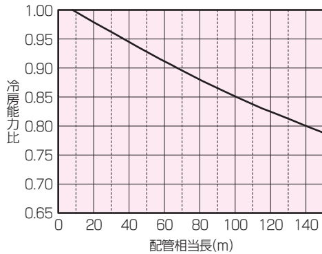
<冷房配管長補正線図>
