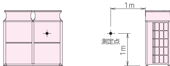
KM-30A
