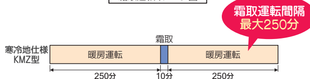
霜取運転イメージ図
