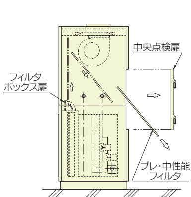
フィルタの取出し
