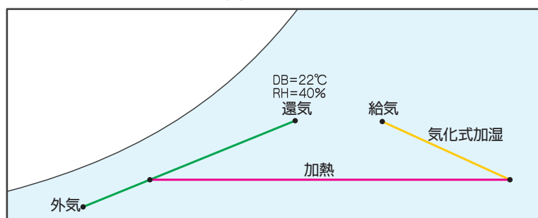
(1) 気化式加湿
