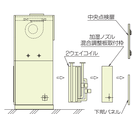
加湿器、コイルの取出し
