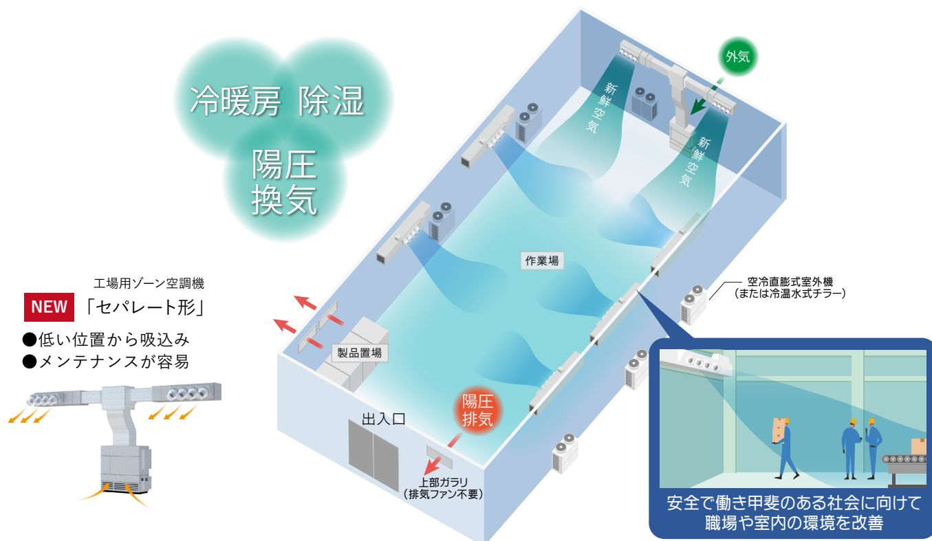
工場用ゾーン空調機
