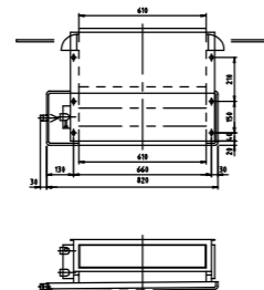
HSR6-300ZF
