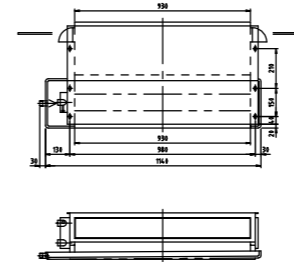
HSR6-600ZF
