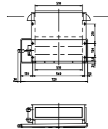
HSR6-200ZF
