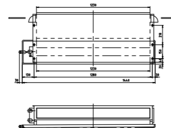
HSR6-800ZF
