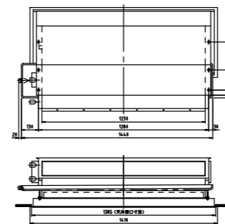
HSR6-800ZBTW2
