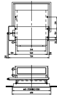
HSR6-200ZBTW2
