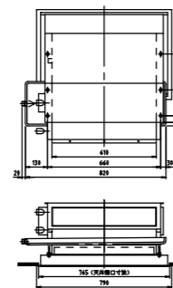
HSR6-300ZBTW2
