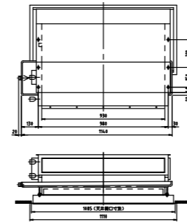
HSR6-600ZBTW2
