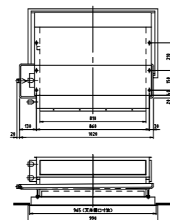
HSR6-400ZBTW2
