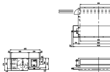
HSR6-400ZF65P2
