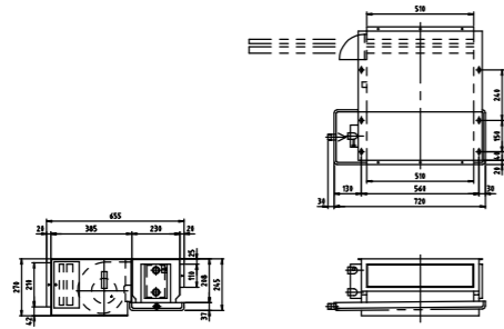
HSR6-200ZF65P2
