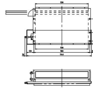
HSR6-600ZF65P2
