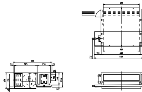
HSR6-300ZF65P2
