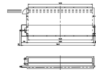
HSR6-1200ZF65P2
