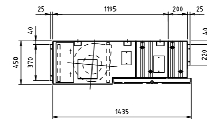
SCH2-4800ZW2
