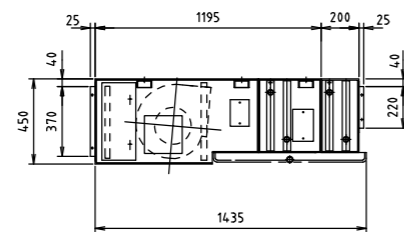
SCH2-2400ZW2
