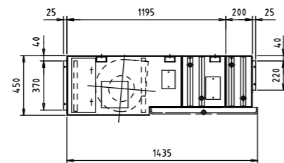
SCH2-1800ZW2
