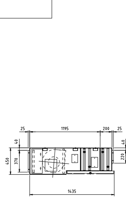
SCH2-1200ZW2
