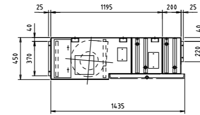
SCH2-3600ZW2
