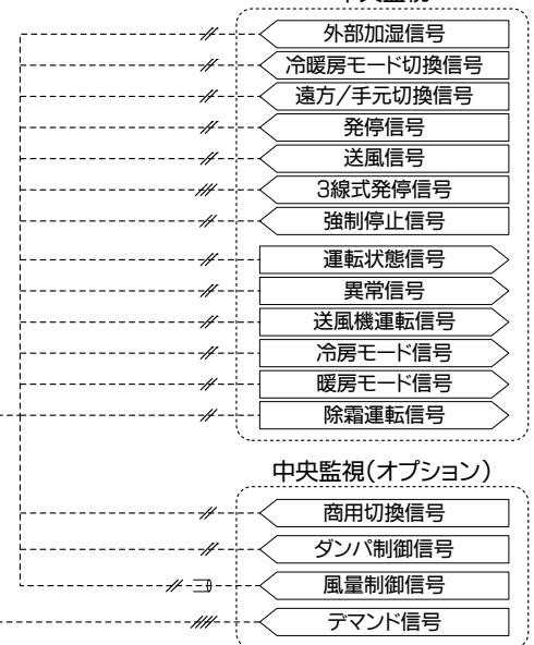
制御盤 オプション入出力仕様表
