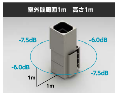
防音防雪フードMOSGHシリーズ 防音効果
