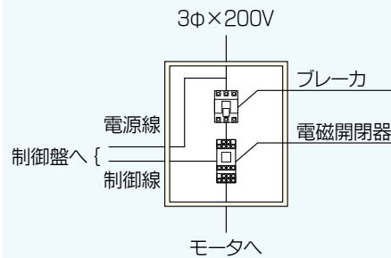
定風量仕様 サーマルボックス
