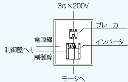
可変風量仕様 インバータボックス
