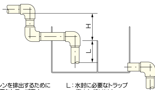
配管トラップの場合
