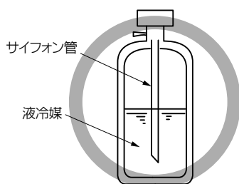
【サイフォン管付きポンベの場合】 立てたまま液冷媒を充てんできる
