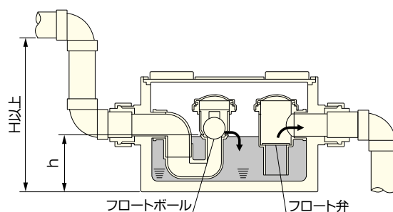
フロートボール式トラップの場合
