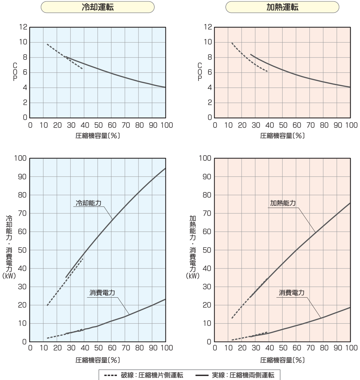
圧縮機容量－能力特性例（RFT-12000S-OA 定格空気条件時）
