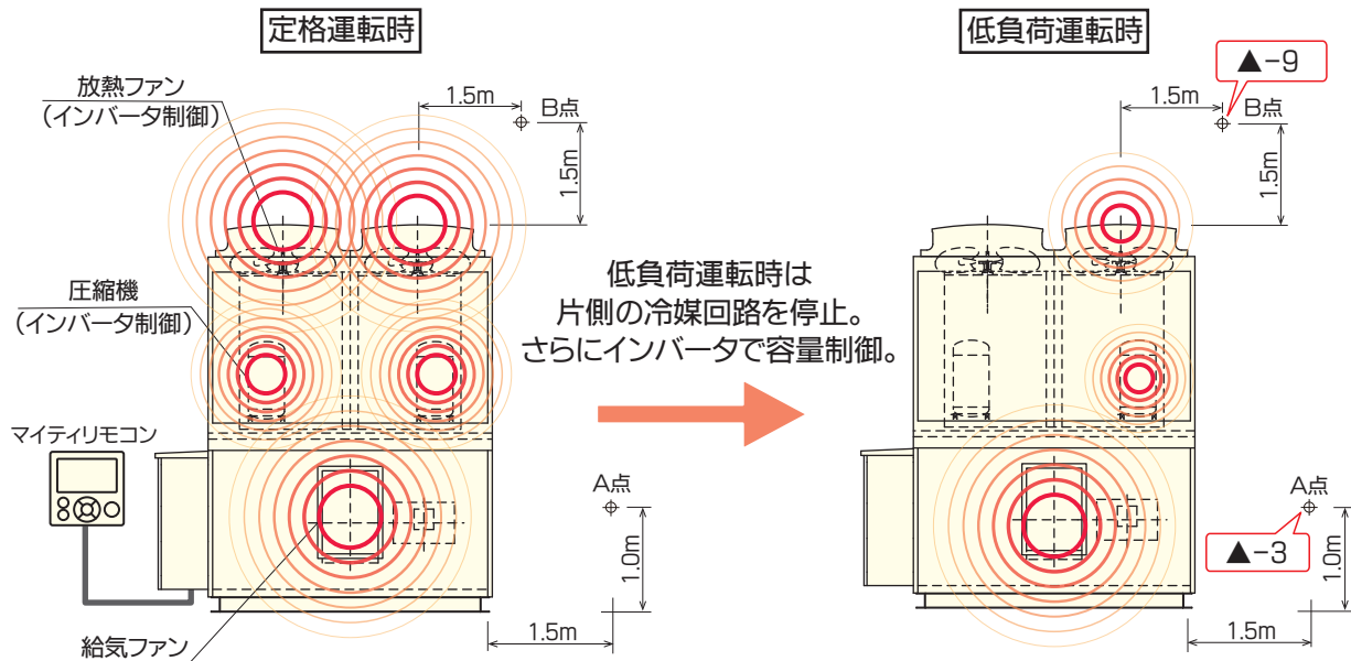
RFT-12000S型 参考騒音値(dB)
