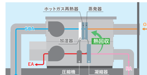
廊下に新鮮外気を給気するBSD-AD型のイメージ
